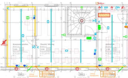
Planausschnitt Obergeschoss
